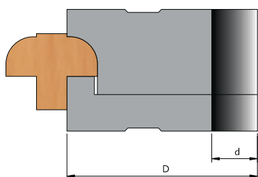
PERFIL 2170.03
