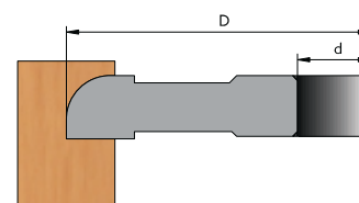
CONTRA-PERFIL 2172.03
